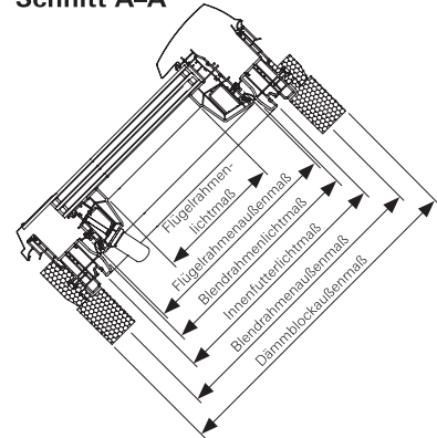
Schnitt A-A
